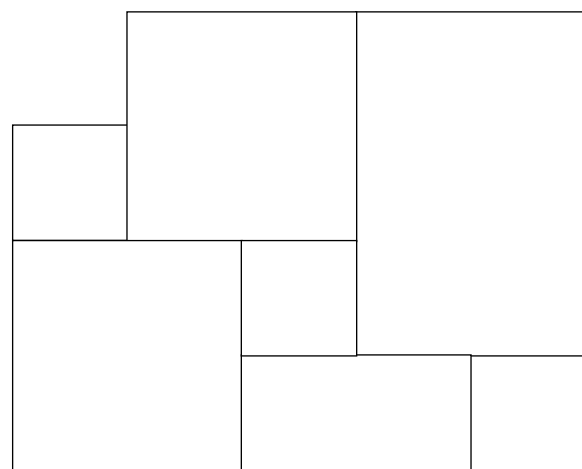
VERSAILLES PATTERN - 8 SF (1) 16X24, (2) 16X16, (1) 8X16, (2) 8X8
