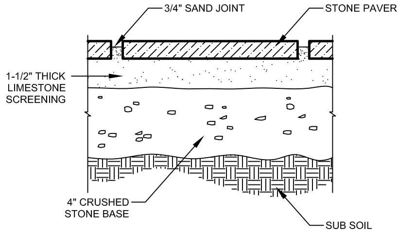
1 STONE PAVERS SET IN SAND BED Scale: 3" = 1'-0"
